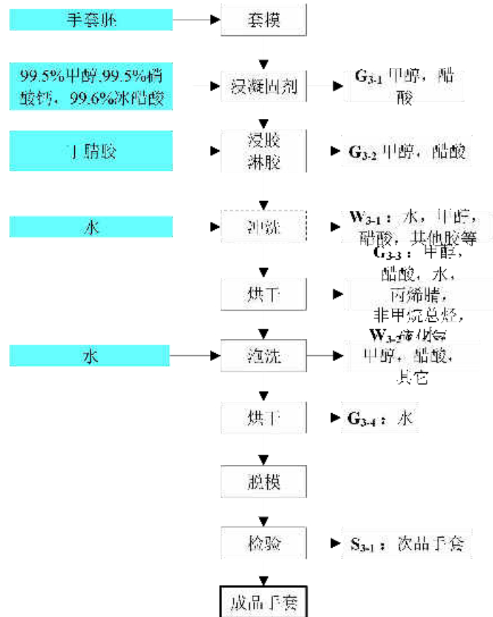
图 4.3-4 生产工艺流程及产物环节图
