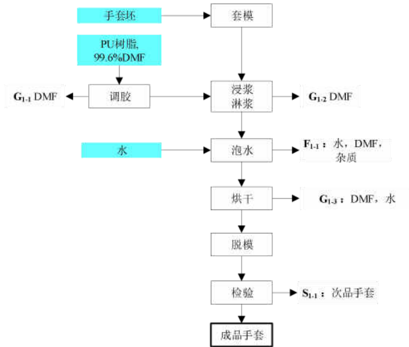
图 4.3-1 生产工艺流程及产污环节图
