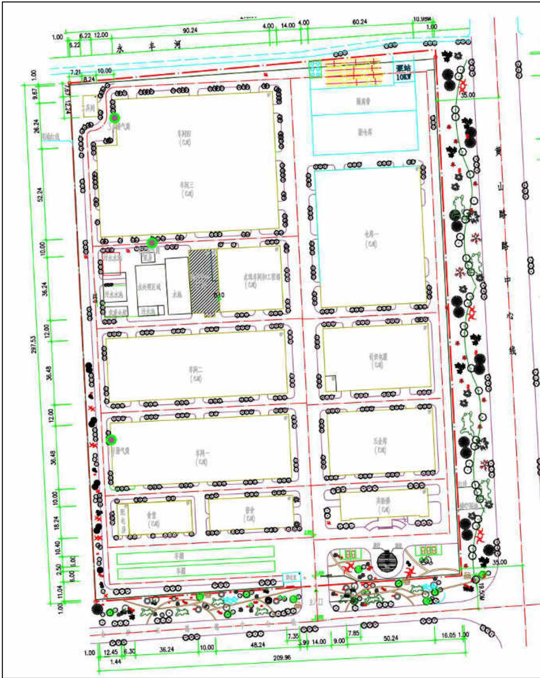
图2.2-1 厂区平面布置图
