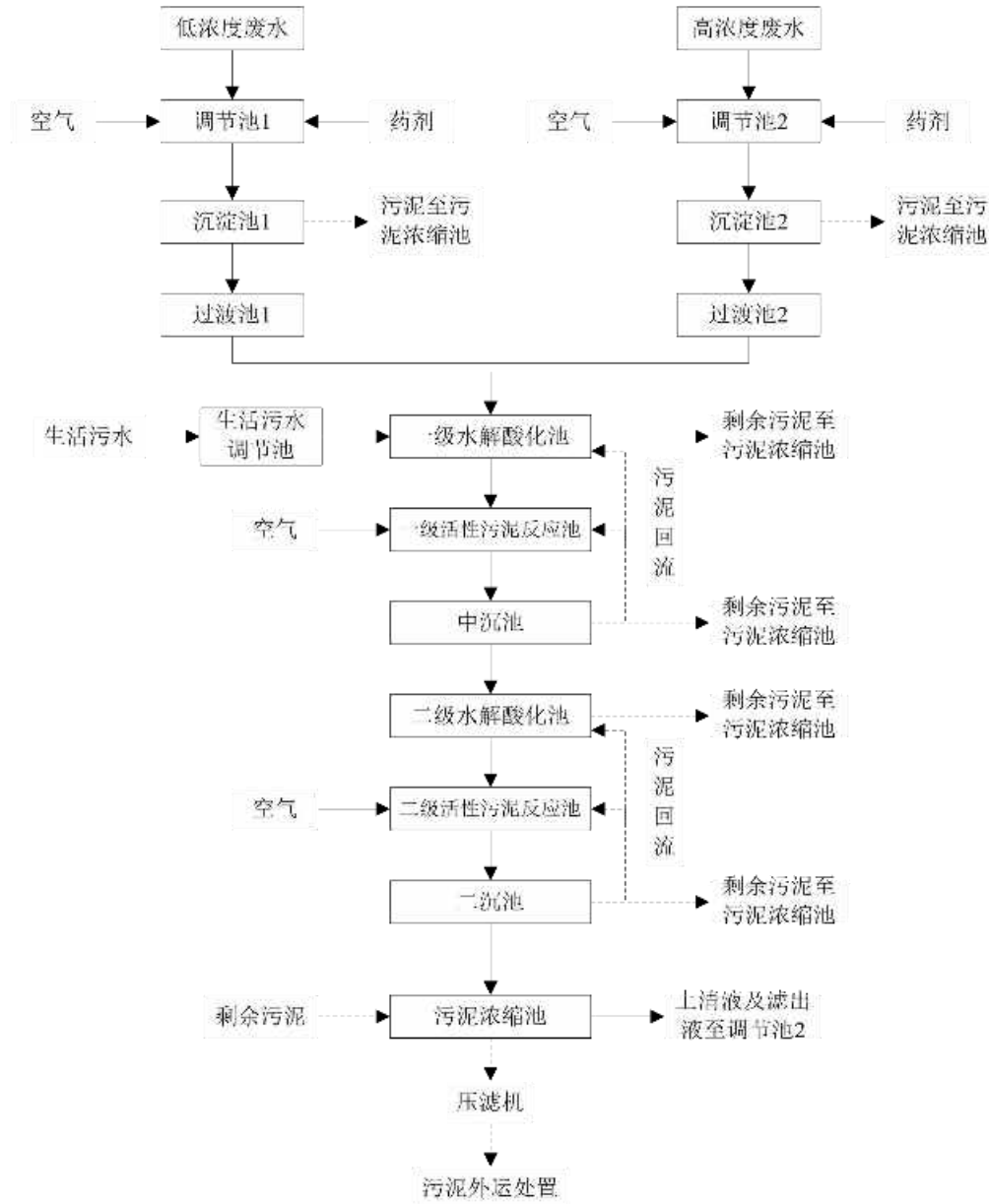
图4.3-7 废水收集流向、处理流程图
