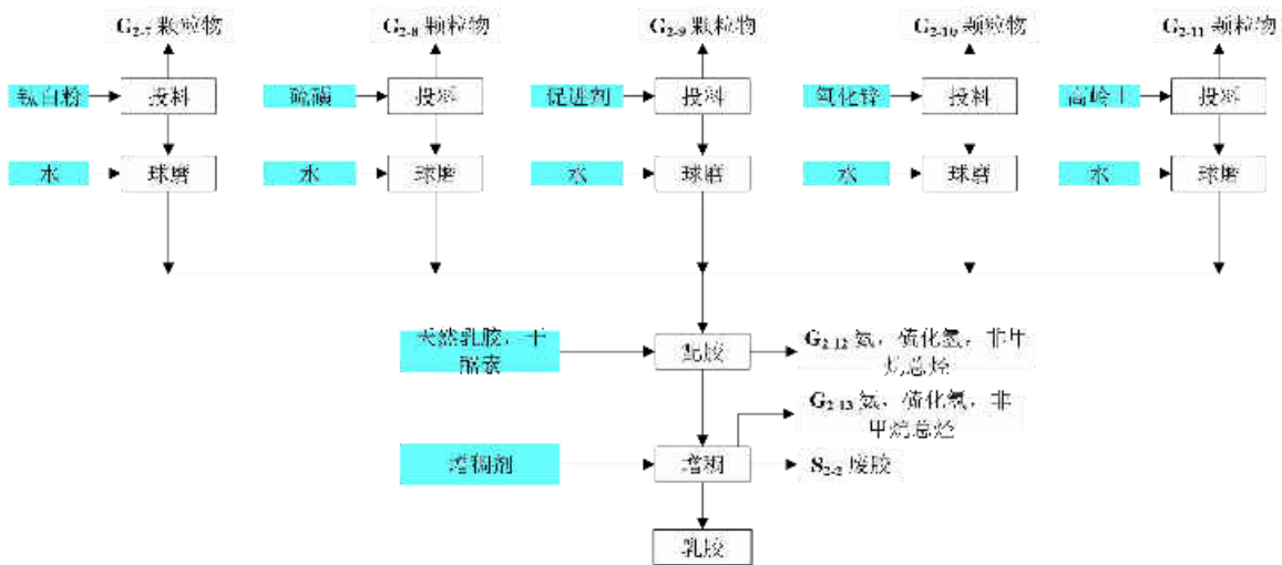
图 4.3-3 乳胶配胶生产工艺流程及产污环节图
