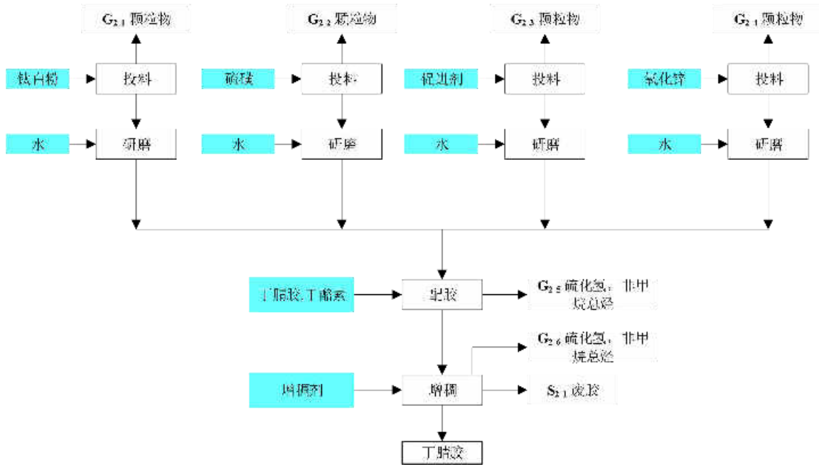
图4.3-2 丁腈胶配胶生产工艺流程及产污环节图
