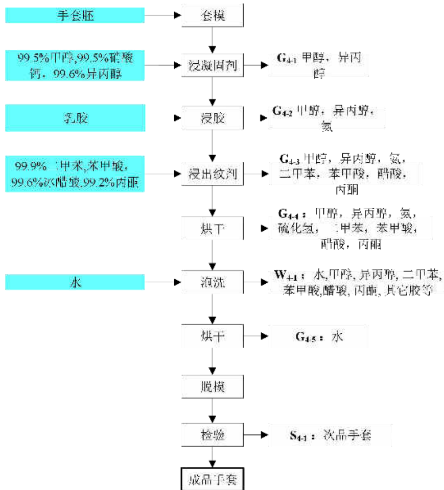
图 4.3-5 生产工艺流程及产物环节图
